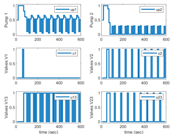
شکل ۸: (ج) ورودی‌های بهینه سیستم
