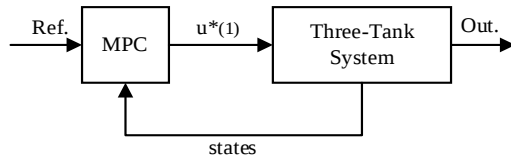
شکل ۴: کنترل کننده پیش‌بین مبتنی بر مدل حلقه بسته
