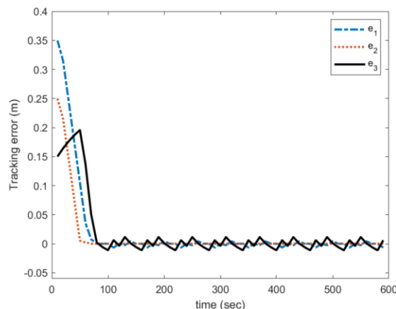
شکل ۸: (ب) خطای ردیابی
