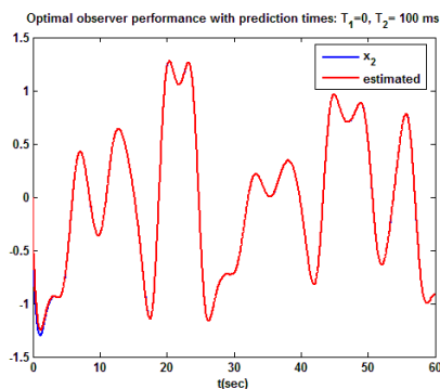
شکل ۴: مسیر حالت سیستم پاندول آشوبناک و تخمین آن توسط روتگر بهینه پیشنهادی
