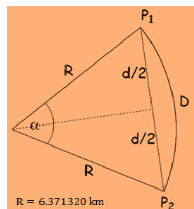
شکل ۶- محاسبه قطاع کره با استفاده از قانون کسینوس و مثلث متساوی الساقین [۸و۶]
