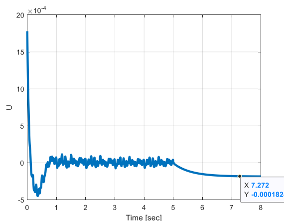
شکل ۵: سیگنال کنترلی
