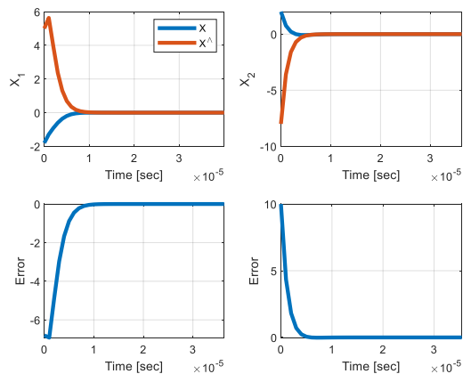
شکل ۸-ب: بزرگنمایی متغیرهای حالت سیستم اصلی، رویکرد و خطای بین آنها
