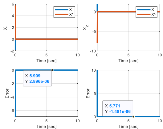
شکل ۸-الف: متغیرهای حالت سیستم اصلی، رویتگر و خطای بین آنها
