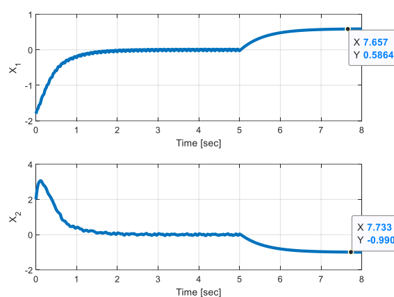
شکل ۴: متغیرهای حالت سیستم
