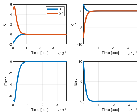
شکل ۸-الف: متغیرهای حالت سیستم اصلی، رویتگر و خطای بین آنها
