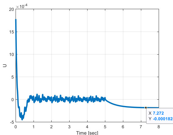
شکل ۵: سیگنال کنترلی
