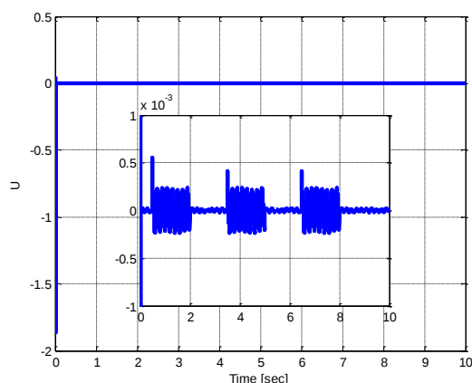
شکل ۱۲-الف: سیگنال کنترلی
