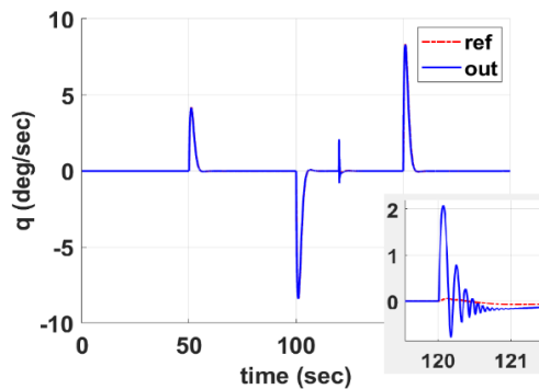
شکل ۲۴: تاریخچه نرخ فراز مطلوب و نرخ فراز خروجی شبیه‌سازی با حلقه درونی دومرحله‌ای در حضور اغتشاش ورودی
