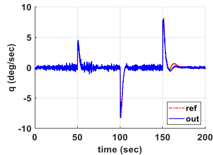
شکل ۲۶: تاریخچه نرخ فراز مطلوب و نرخ فراز خروجی شبیه‌سازی با حلقه درونی دومرحله‌ای در حضور نویز اندازه‌گیری
