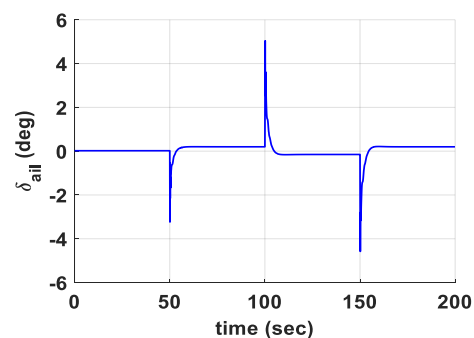
شکل ۱۶: تاریخچه ورودی کنترلی شپهر
