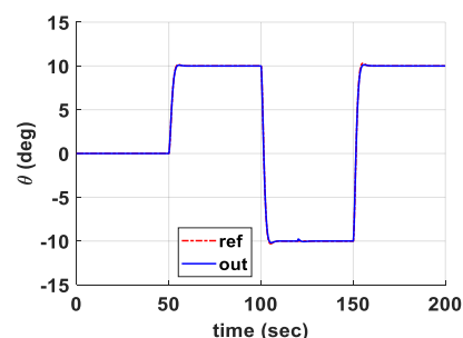
شکل ۲۸: تاریخچه زاویه فراز مطلوب و زاویه فراز خروجی شبیه‌سازی با حلقه درونی دومرحله‌ای در حضور اغتشاش ورودی
