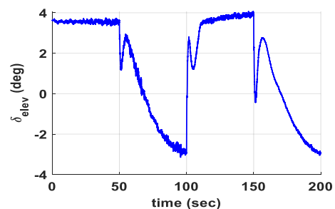
شکل ۲۷: تاریخچه ورودی کنترلی بالابر با حلقه درونی دومرحله‌ای در حضور نویز اندازه‌گیری
