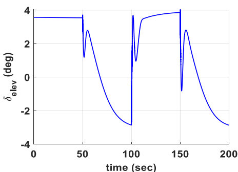
شکل ۱۹: تاریخچه ورودی کنترلی بالابر با حلقه درونی دومرحله‌ای
