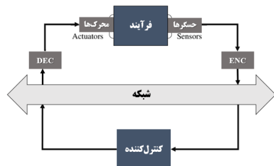
شکل ۳: یک ساختار نوعی برای NCS
