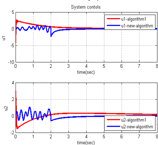
شکل ۱۴: سیگنال های کنترلی وارد شده به سیستم دوخطی در طول فرآیند یادگیری و بعد از آن
