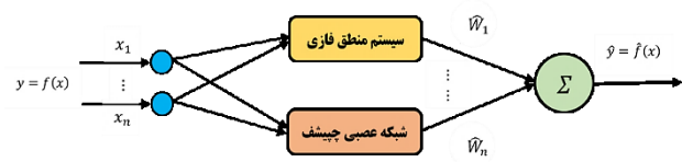
شکل ۲: ساختار موازی شبکه عصبی چشیف فازی پیشنهادی
