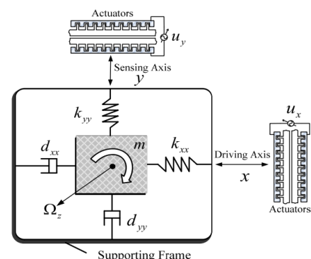
شکل ۳: ساختار ژيروسکوپ میکروالکترومکانیکی [۱]
