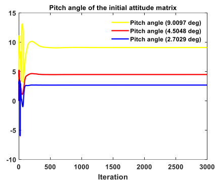
شکل ۸: نمایی از تخمین زاویه فراز در ماتریس وضعیت اولیه در شرایط
