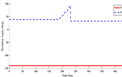
ج) تغییرات زاویه سر دو پهپاد
