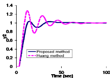
شکل ۹. مقایسه پاسخهای خروجی از سیستم کنترل حلقه دوم، به هنگام تغییر پله ای در مقدار مقرر حلقه اول
