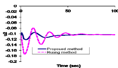
شکل ۱۱. مقایسه پاسخهای خروجی از سیستم کنترل حلقه دوم، به هنگام تغییر پله ای واحد در مقدار مقرر حلقه اول
