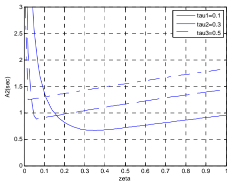
شکل ۸: شرط پایداری A_2 بر حسب \zeta به ازای K_1 = 0.5, \alpha = 0 و مقادیر مختلف \tau_1 و K_2 = 4 و \omega_n = 10
