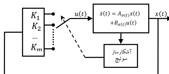
شکل ۱: نمایش شماتیک پایدارسازی سیستم سوئیچینگ خطی با استفاده از فیدبک حالت
