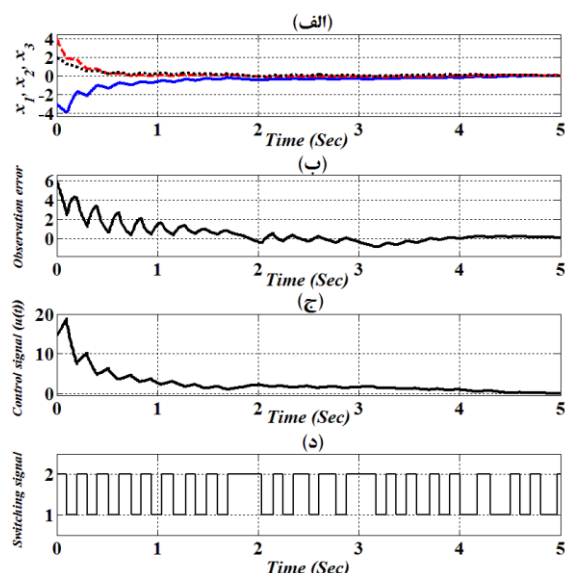
شکل ۴: (الف) حالت‌های سیستم سوئیچینگ خطی پایداری شده با استفاده از فیدبک حالت مبتنی بر روتگر، (ب) خطای روتگر حالت e(t) = (y(t) - C_{\sigma(t)}\hat{x}(t)) ، (ج) سیگنال کنترلی u(t) = K_{\sigma(t)}\hat{x}(t) و (د) سیگنال سوئیچ با حداقل زمان اقامت ۰/۱ ثانیه برای سیستم سوئیچینگ مثال ۲ و پارامترهای a = 5.4 ، b = 5.7 و c = 4.5 .
