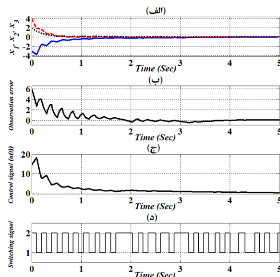
شکل ۵: (الف) حالت‌های سیستم حلقه بسته پایداری شده با استفاده از فیدبک حالت مبتنی بر روتگر، (ب) خطای روتگر حالت e(t) = (y(t) - C_{\sigma(t)}\hat{x}(t)) ، (ج) سیگنال کنترلی u(t) = K_{\sigma(t)}\hat{x}(t) و (د) سیگنال سوئیچ با حداقل زمان اقامت ۰/۱ ثانیه، برای سیستم سوئیچینگ مثال ۲ و پارامترهای a = 6 ، b = 5 و c = 4 .
