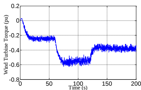
شکل ۱۲ - گشتاور توربین بادی
