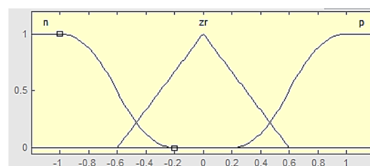
شکل ۷: سیگنال مشتق خطا
