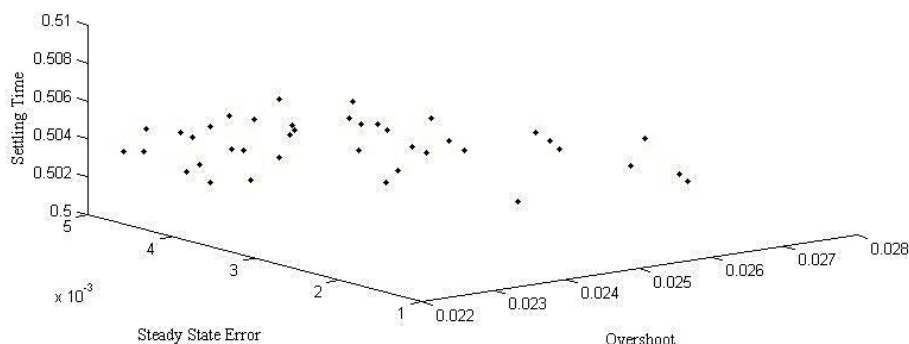
شکل ۹: Pareto front
