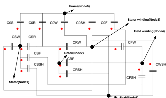
شکل ۵: خازنهای پارازیتی متقابل شش گره ژنراتور سنکرون
