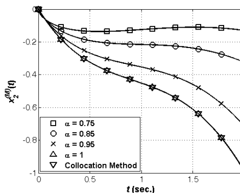
شکل ۵: نمودارهای حالت زیر-بهینه مرتبه پنج x_2^{(5)}(t) محاسبه شده توسط روش سری مودال به ازای مقادیر مختلف \alpha به همراه روش کولوکیشن (مثال ۲).
