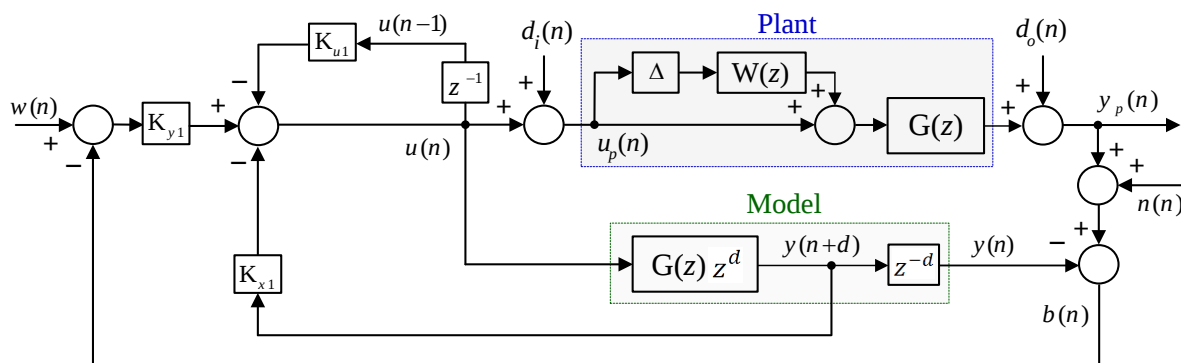
شکل ۲: بلوک دیاگرام معادل ساختار کنتری، ارائه شده در این مقاله به صورت اسمیت.
