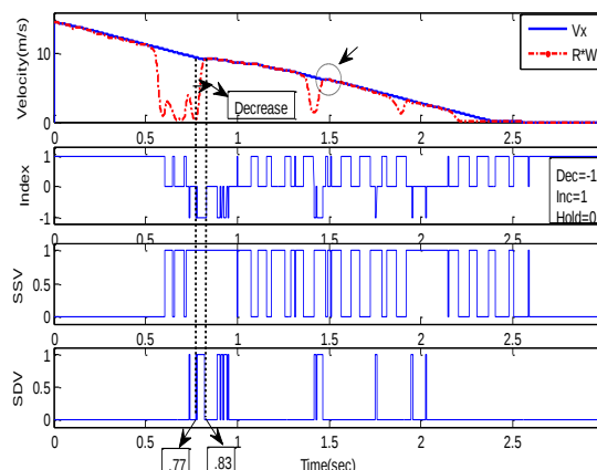
شکل ۳: نقاط قله سرعت خطی چرخ و برابری سرعت طولی خودرو با سرعت خطی چرخ ها در نقاط مشخص شده و ناحیه کاهش فشار پشت کالیپر (معادل شاخص -1 ) و وضعیت شیرهای برقی ورودی و خروجی و زمان مورد نیاز سیستم برای رسیدن به نقطه قله سرعت خطی چرخ
