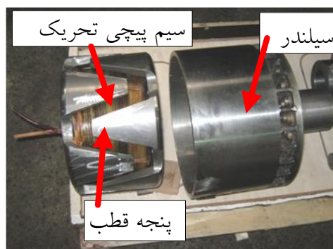
شکل ۲: ساختار دینامومتر جریان فوکو قطب پنجه‌ای [۳]
