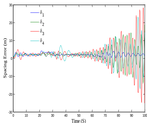
شکل ۹: ناپایداری رشته‌ای و داخلی سیستم در سناریو ۴
