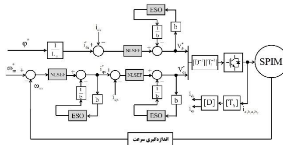
شکل ۳: نمودار کنترل برداری موتور القایی شش فازه در حالت استفاده از ADRC
