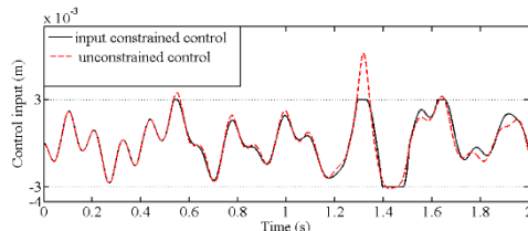
شکل ۱۰: ورودی کنترلی (جابه‌جایی قرقره شیر هیدرولیک) در سیستم تعلیق فعال نامقید و مقید
