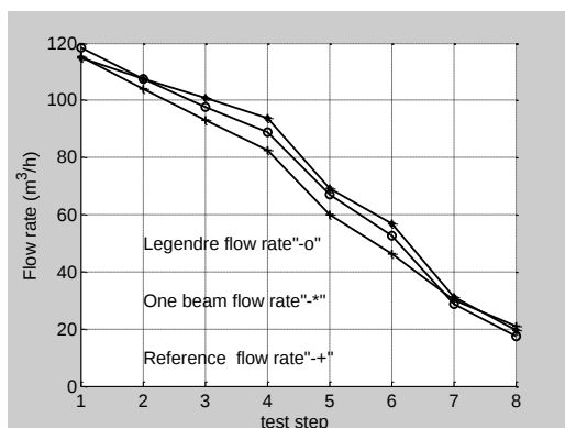
شکل ۹- نتایج اندازه گیری نرخ سیال در دی سنس های تک مسیره و چهار مسیره و مقایسه آنها با مقدار مرجع
