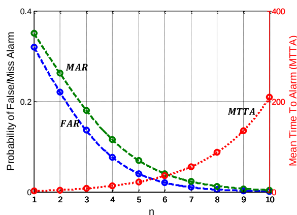
شکل ۷: تأثیر افزایش تعداد تأخیر بر شاخص های سیستم هشدار.
