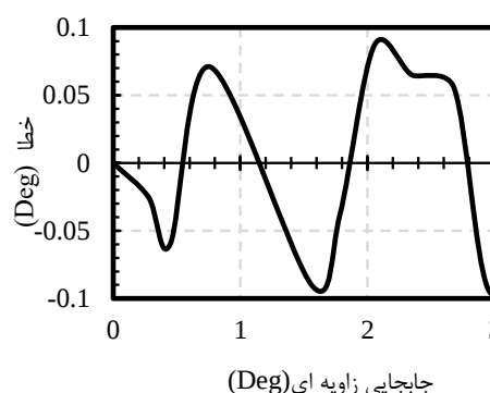
شکل ۱۰: نمودار خطا خروجی انکودر به ازای ۱۰ و ۳ درجه جایابی
