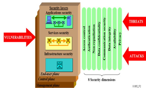
شکل ۳: معماری امنیت از دید استاندارد ITU-T X.805 [۲۸]
