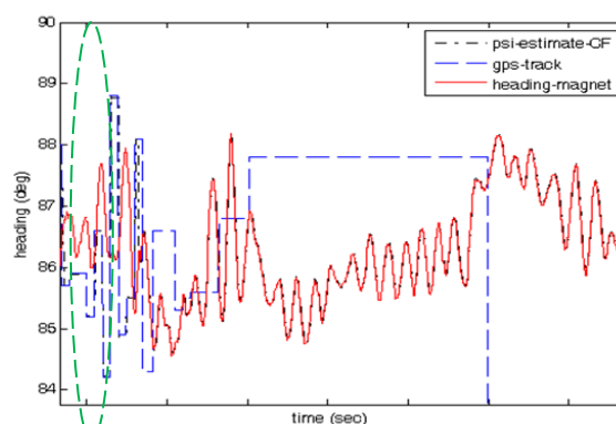
شکل ۱۰- تخمین زاویه سمت با سوئیچ از GPS به مغناطیس سنچ در فاز حرکت زیر سطحی
