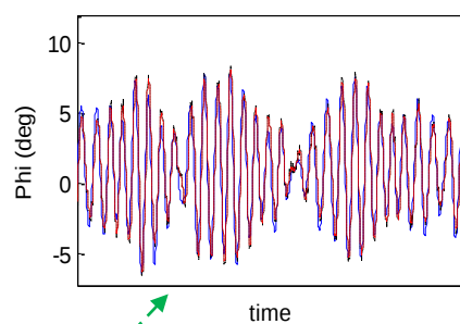
شکل ۷- مقدار واقعی زاویه فراز و تخمین آن با فیلتر تکمیلی و کالمن
