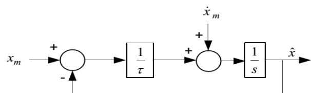
شکل ۳- فیلتر تکمیلی غیرمستقیم (۲و۱)
