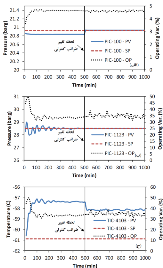
شکل ۴: تغییرات مرتبط با کنترل کننده‌های اصلی در حالت خوراک طراحی:
