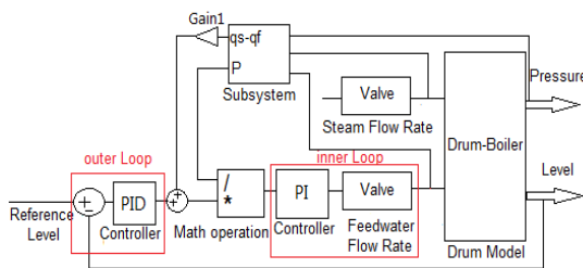
شکل ۵: منطق پیشنهادی کنترل سطح درام
