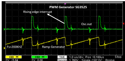
شکل (۱۱) - سیگنال Osc.out و موج دنداناره آره ای، تولید شده توسط SG3525
