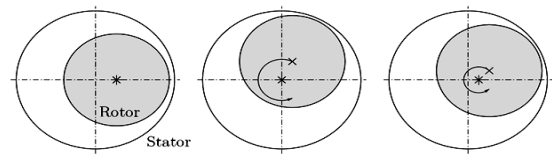
شکل ۳: شماتیک از گریز مرکزهای استاتیکی، دینامیکی و مختلط. * مرکز چرخشی رتور و × مرکز هندسی رتور تعریف می شوند
