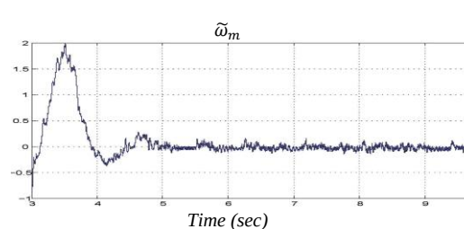
شکل ۹: عملکرد سیستم FTC در حضور خطای مکانیکی استاتور
