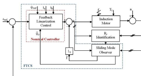
شکل ۵: سیستم کنترل تحمل پذیر خطا برای موتور القایی سه فاز.
