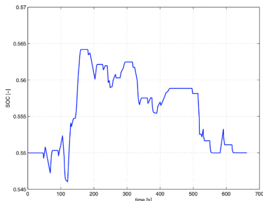
شکل ۱۶: نمودار SOC در روش پیشنهادی
