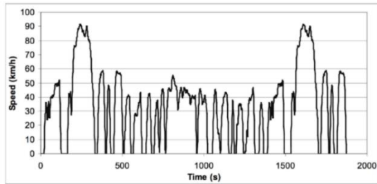
شکل 9: نمودار سرعت-زمان سیکل رانندگی FTP-75 (استرالیا)
