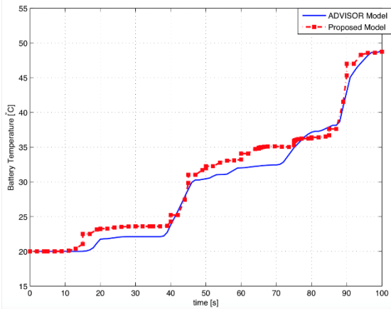
شکل 8: راستی آزمایی مدل گرمایی باتری
