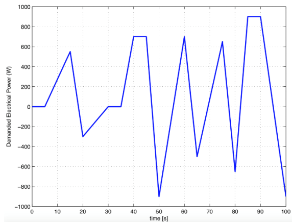
شکل 7: سیگنال توان الکتریکی درخواستی برای راستی آزمایی مدل
