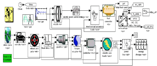
شکل 6: مدل یک خودروی هیبرید الکتریکی موازی در ADVISOR
