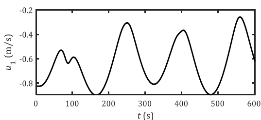
شکل ۱۱: اولین ورودی کنترلی سینماتیکی برای شرایط اولیه I.C. 1 در حرکت رو به عقب
