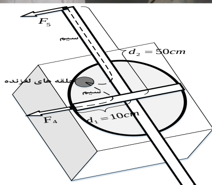
شکل ۵: موتور استفاده شده برای شبیه‌سازی حرکت غلت پرتابه
