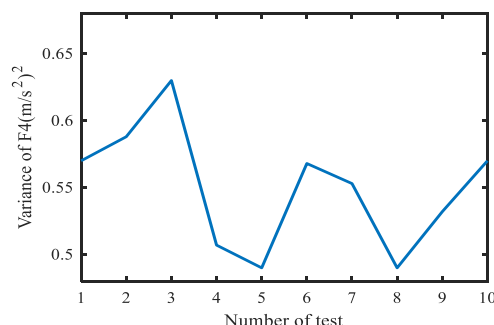
شکل ۷: واریانس حسگر F_4 برای سرعت ثابت
