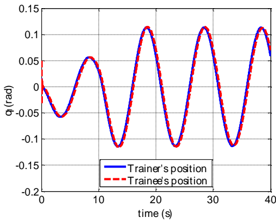
شکل ۶ موقعیت مفصل اول ربات با اعمال کنترل کننده پیشنهادی
