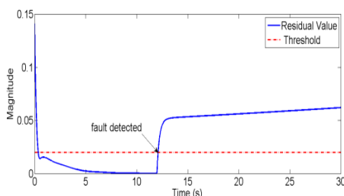
شکل (۳) تشخیص وقوع عیب سنسوری در لحظه ۱۲ برای شرایط اولیه
