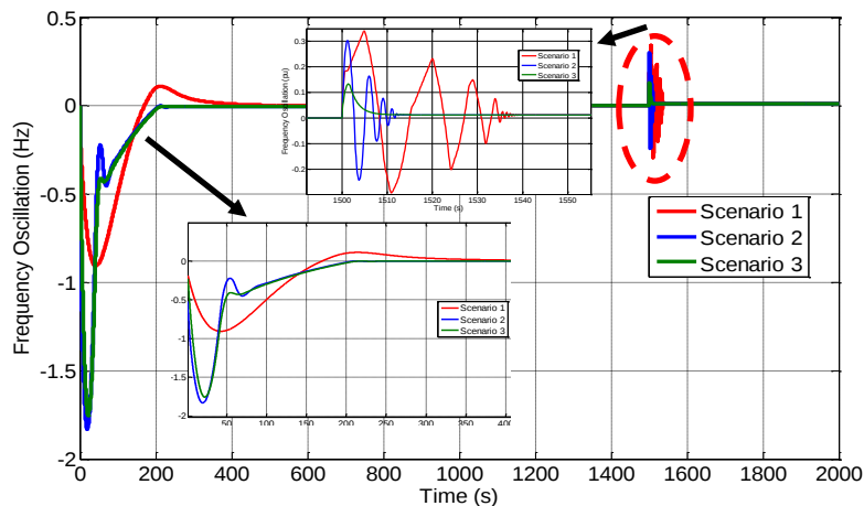
شکل ۹: مقایسه رفتار فرکانسی ریز شبکه در سناریوهای مختلف شبیه سازی
