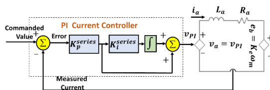
شکل ۶: حلقه کنترل کننده جریان
