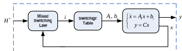
شکل ۲: توصیف ساختار کلاس هابیرید DPWA
