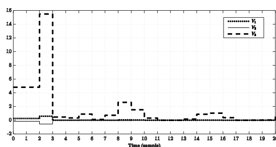
شکل ۴: مقادیر متغیرهای \hat{V}_1(\tilde{x}_t) ، \hat{V}_2(\tilde{x}_t) و \hat{V}_3(\tilde{x}_t) به ازای k = 3
