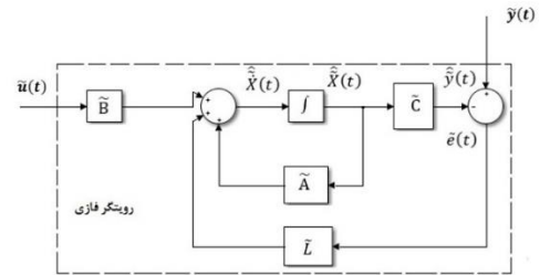
شکل ۳: شمای کلی رویتگر خطی فازی
