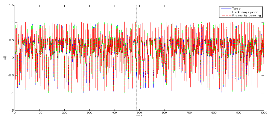
شکل ۱۱- نمودار شناسایی سری زمانی آشوبی هنون توسط شبکه عصبی راف بهبود یافته با ۳ نرون با یادگیری احتمالاتی
