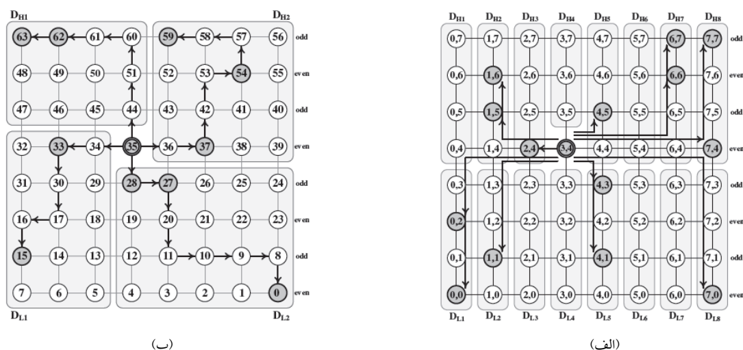
شکل ۱: مثال‌هایی از الگوریتم‌های چندپخشی مبتنی بر مسیر و بر پایه بخش‌بندی (الف) ستونی، (ب) چندمسیره
