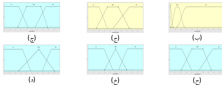
شکل ۲: الف) سیستم فازی. ب) تابع عضویت ورودی Fbest ب) تابع عضویت ورودی Iteration ج) تابع عضویت خروجی C1 ج) تابع عضویت خروجی C2 د) تابع عضویت خروجی W ج) تابع عضویت خروجی Popsiz.
